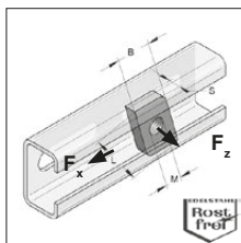
Płytki z otworem gwintowanym
