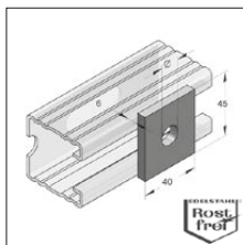
Płytki z otworem
